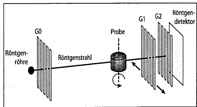
Aufbau eines Talbot-Gitterinterferometers zur Phasenkontrastmessung. Lesen Sie mehr ab ► Seite 16
