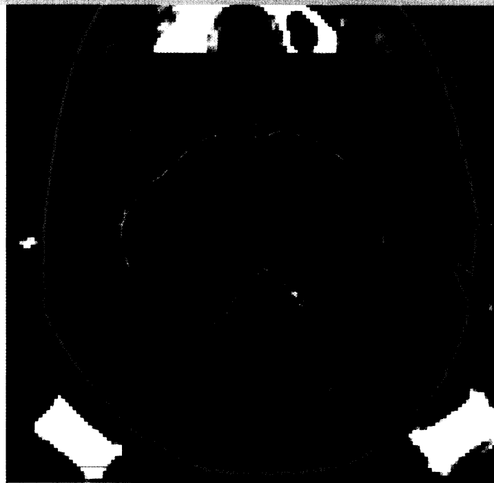
Protonenbestrahlung
