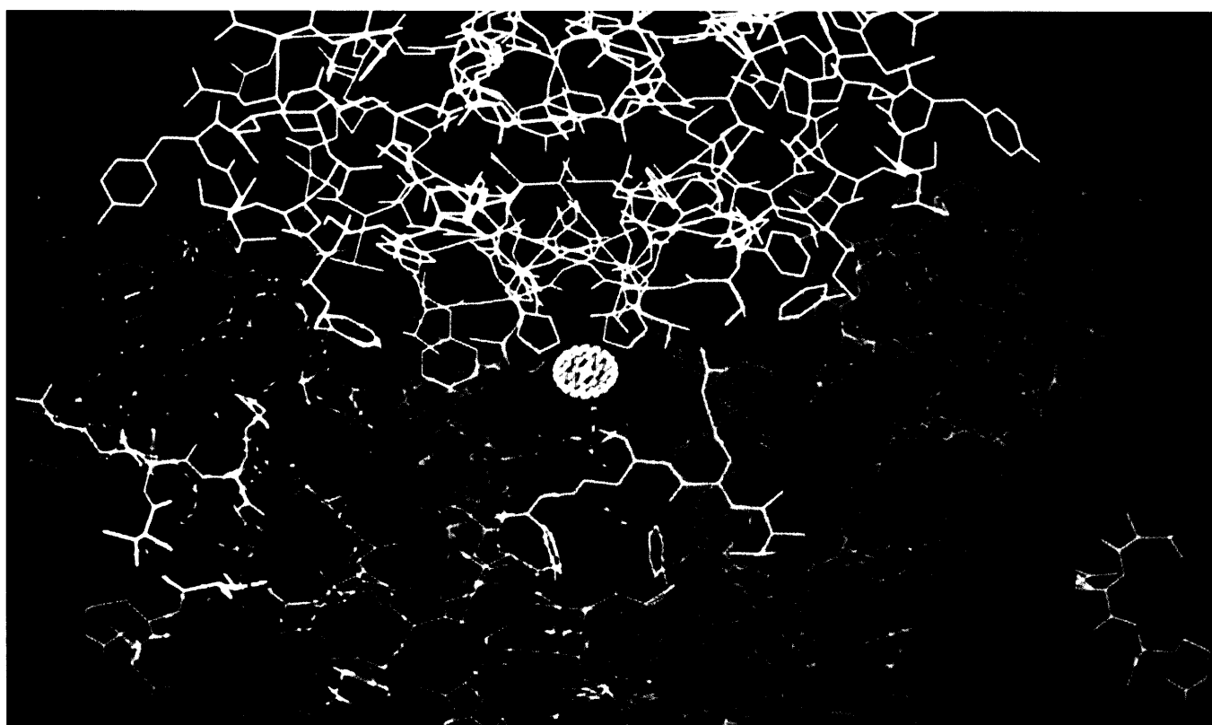
Molekularstruktur eines Glargins
