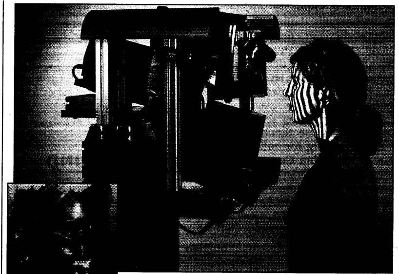
G-Scan-Meß-System, mit dem sich berührungslos ein 3D-Bild erzeugen läßt. Foto: Fraunhofer-Institut, Jena
