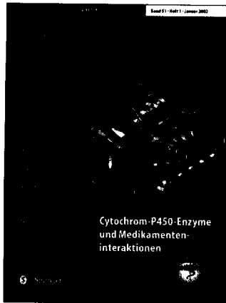
Titelbild: Strukturmodell eines Cytochrom P450-Enzyms mit eingebauten Häm-Eisen-Komplex (Quelle: Dr. Matthias Schwab, Dr. Margarete-Fischer-Bosch Institut für Klinische Pharmakologie, Auerbachstrasse 112, 70376 Stuttgart). Gestaltung: de'blik, Berlin
