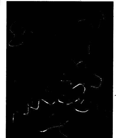
Computermodell des PXR-Rezeptormoleküls (rot) mit dem Modell eines Lipidsenkers in der Mitte des Bildes. Foto: Watkins, Redinbo/UNC
